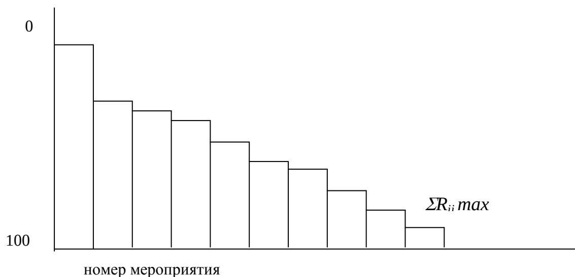
Рис. 1. Диаграмма рангов
